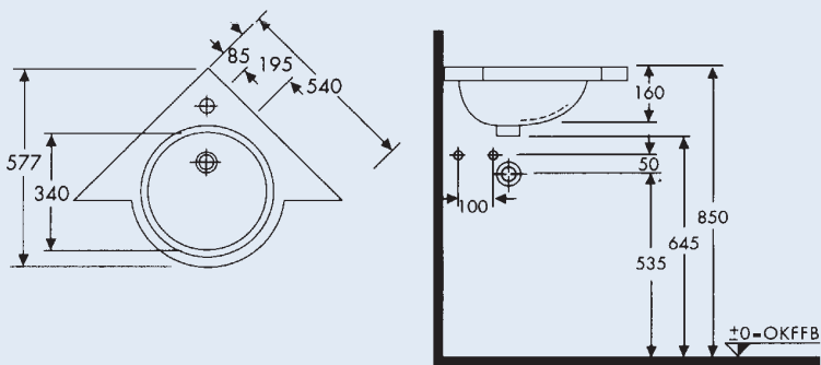
Eck-Einzel-Waschtisch
